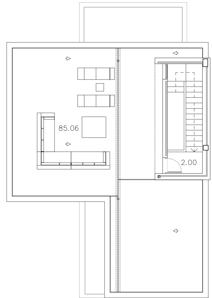
PLANTA CUBIERTA
